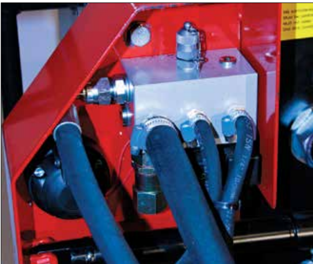
Elektro-hydraulisk sentral for pakke «super»
